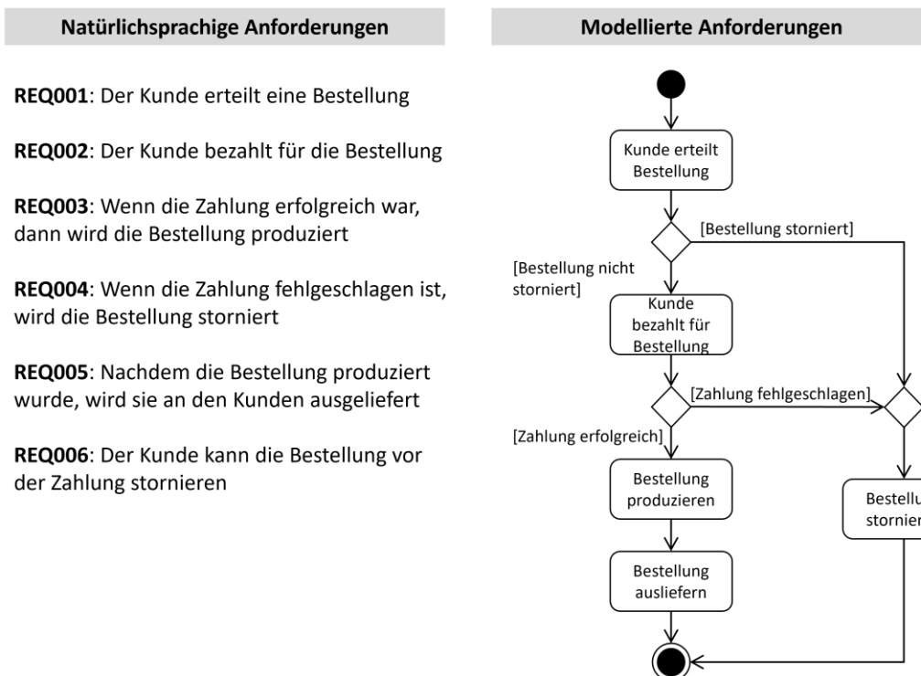
Abbildung 3.2 Textuelle Anforderungen versus modellierte Anforderungen
