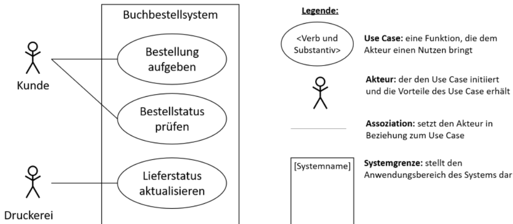
Abbildung 3.6 Beispiel für ein Kontextdiagramm unter Anwendung eines UML-Use-Case-Diagramms
